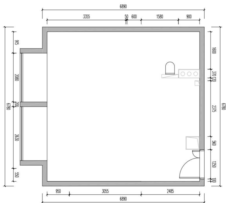
一室一厅户型图
