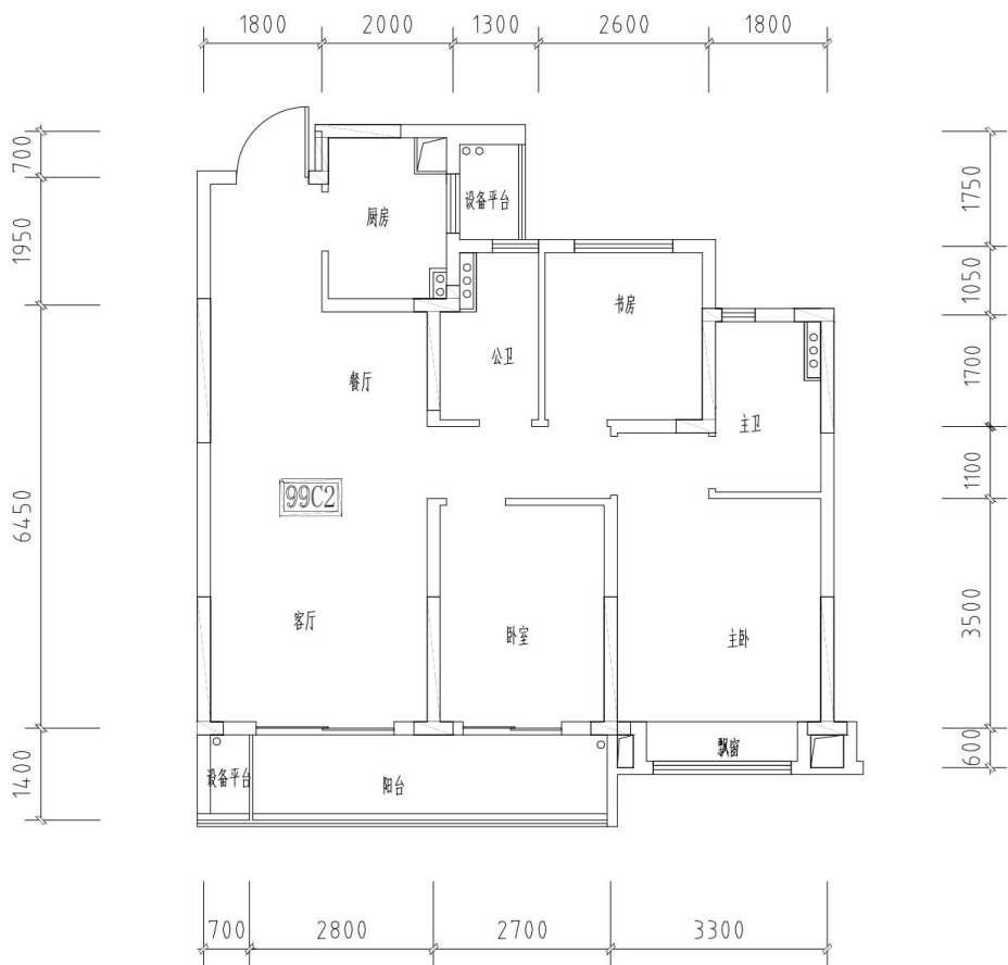
三室一厅户型图
